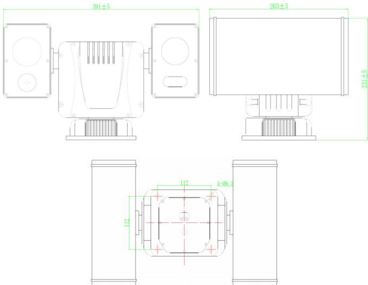
图 3.1 热成像双光谱 T 型摄像机机械尺寸图 (单位: mm)
