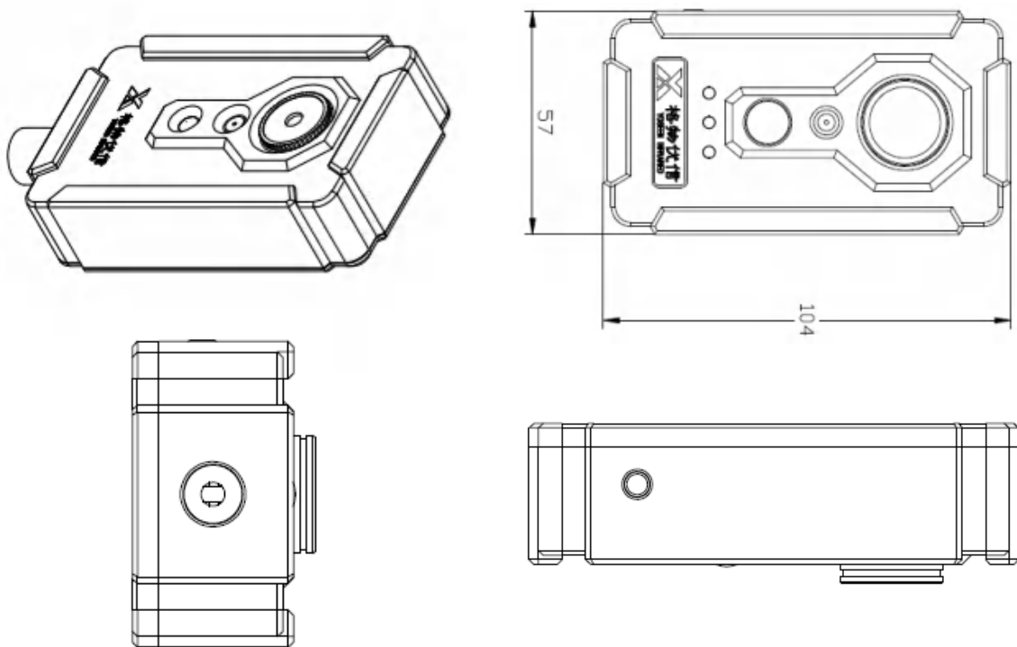
图 3.2 热成像双光谱卡片式摄像机机械尺寸图（单位：mm）
