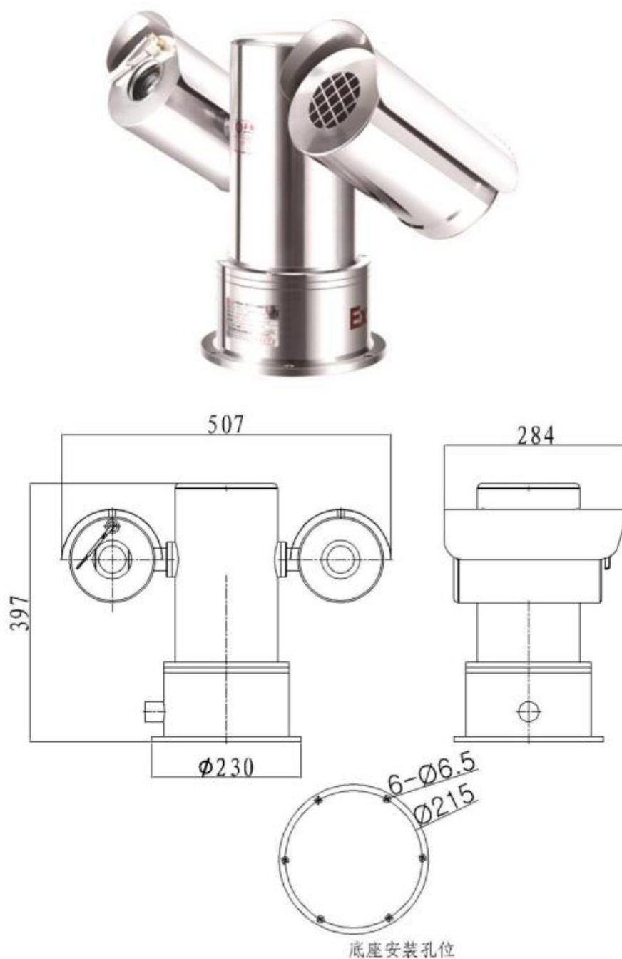
图 3.1 热成像双光谱防爆型摄像机外观及尺寸(单位: mm)
