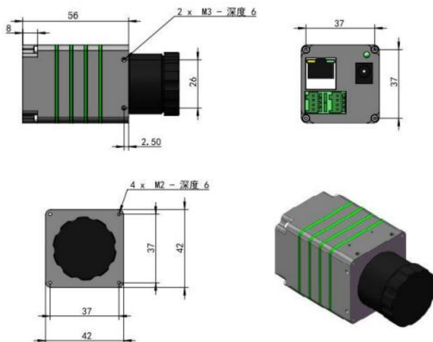
图 3.1 网络型产品外观尺寸(单位: mm)
