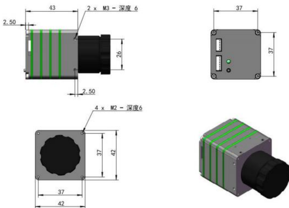
图 3.2 模拟型产品外观尺寸(单位: mm)
