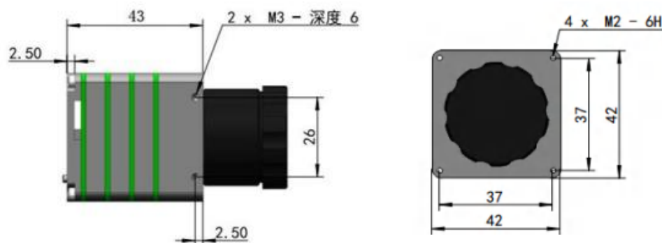
图 4.3 机械安装孔尺寸(单位: mm)
