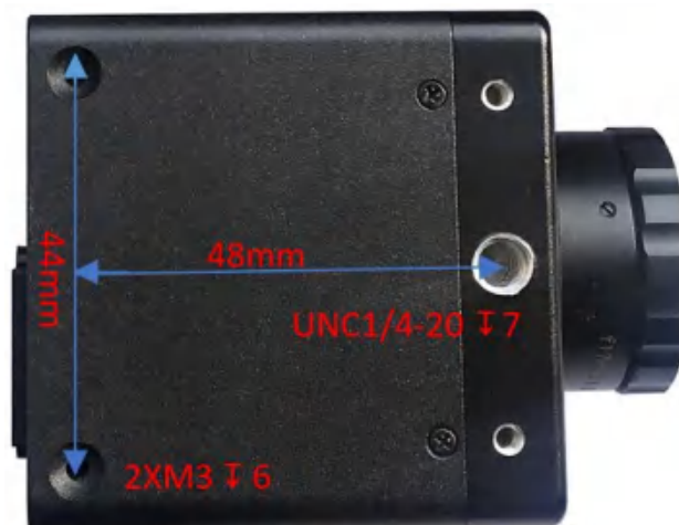
图 3.2 机械安装孔尺寸
